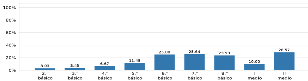
Gráfico 1.1. Porcentaje de estudiantes que demostró avances en los niveles de logro en OA priorizados en Lectura
